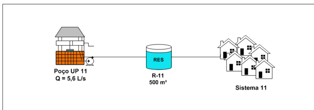
Figura 24 – Croqui Sistema 11.
