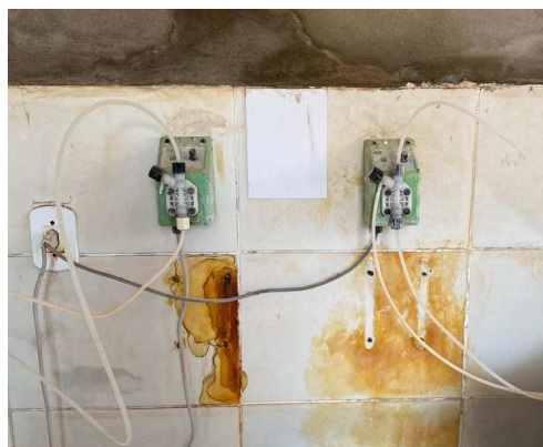
Figura 39 – Bombas dosadoras de cloro e flúor.
