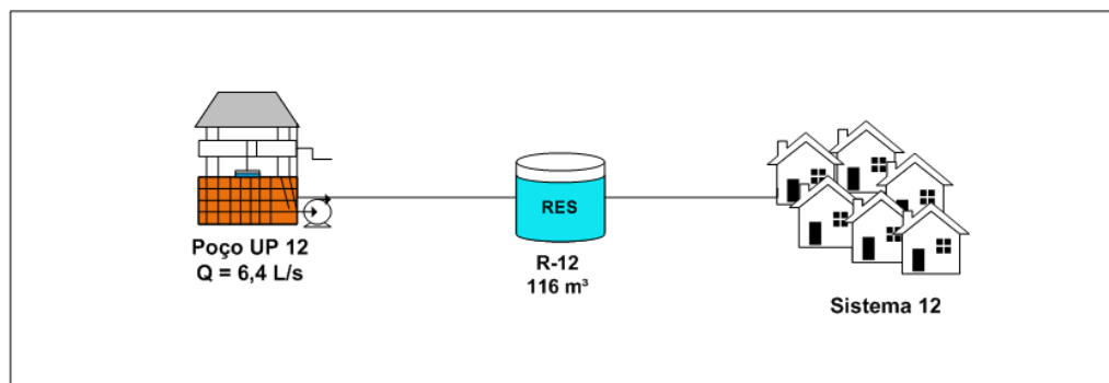
Figura 25 – Croqui Sistema 12.
