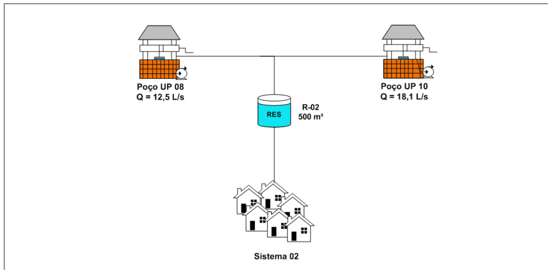
Figura 22 – Croqui Sistema 02.
