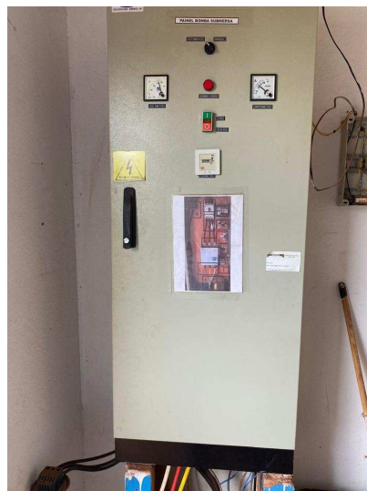
Figura 58 – Painel de comando.
