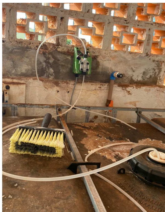
Figura 52 – Bomba dosadora de cloro.
