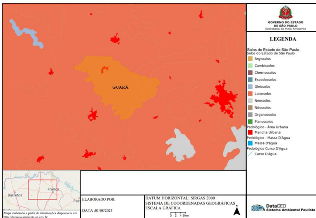
Figura 5 - Classificação de solos da região de Guará.
