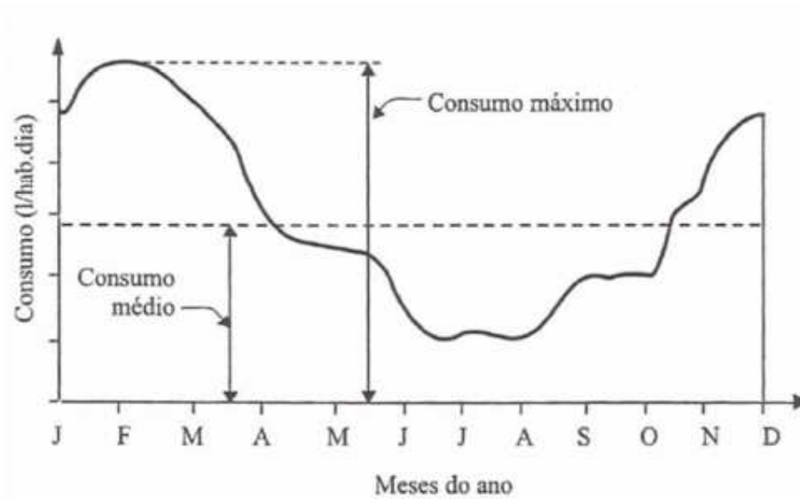
Figura 142 - Variação do Consumo Durante 1 ano (SAA).
