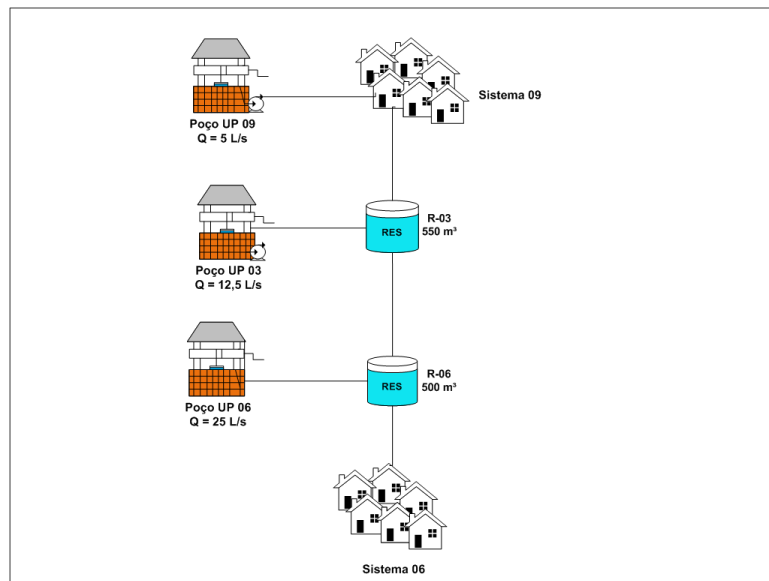
Figura 23 – Croqui Sistema 06.
